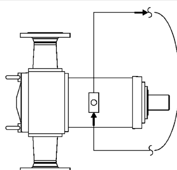
Plan 54 (suministro de presión de bloqueo externo)
