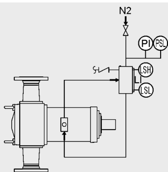
Plano 53 A (sistema de termosifón)
