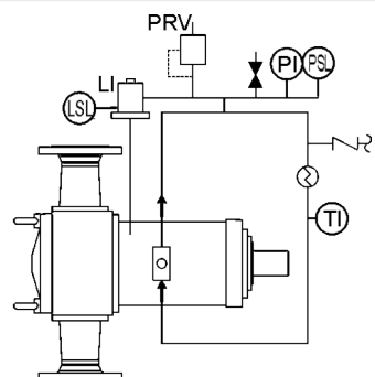
Plan 53 C (sistema acumulador de pistón)
