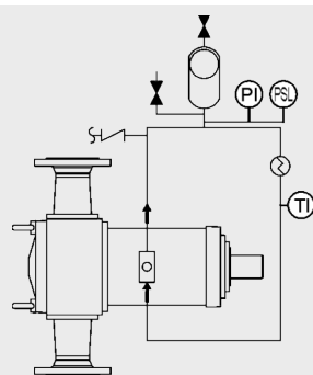
Plano 53 B (sistema acumulador de vejiga)
