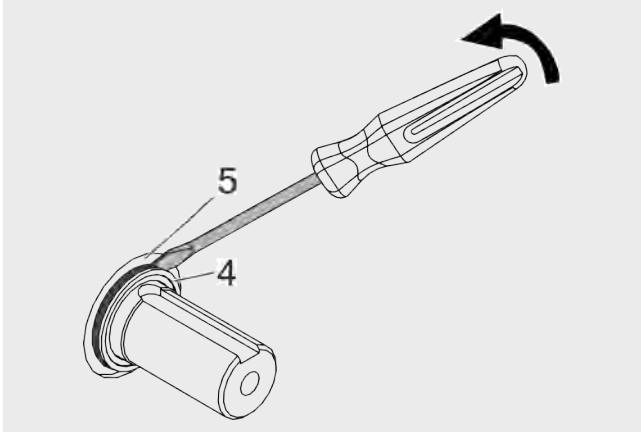
Casquillos estacionarios (5) - retirar los anillos de deslizamiento (4)
