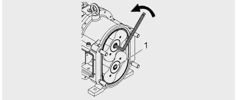
1 Tornillo de sujeción del lóbulo
